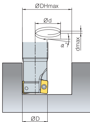
2. Fresatura elicoidale per fori ciechi
