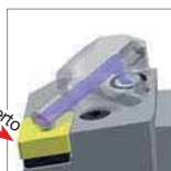
Direzione del getto direttamente sull'inserto
