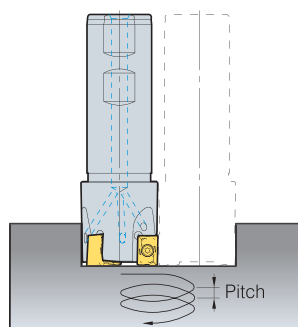
2. Fresatura elicoidale per esecuzione di un foro cieco
