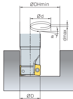
2. Fresatura elicoidale per fori passanti
